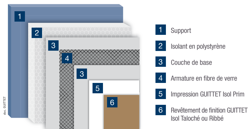
PPG ISOL POUDRE, système à couche de base en poudre à base de ciment
