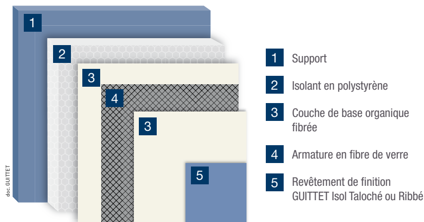
PPG ISOL PAE, système à couche de base organique fibrée
