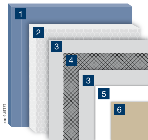
PPG ISOL, système à couche de base pâte+ciment
