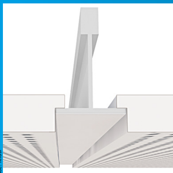
bord E+ ossature semi-apparente
