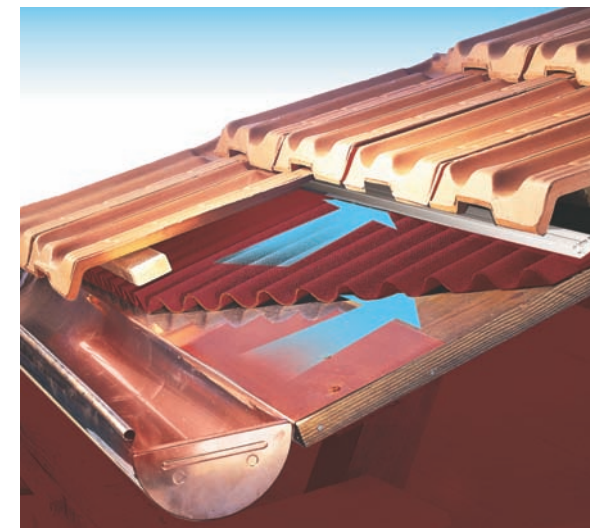
FLEXOUTUILE® permet la ventilation de la toiture grâce à un double flux d'air.
