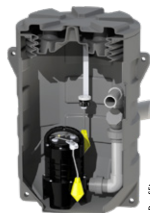
SANIFOS 280 avec alarme filaire en option
